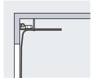
Kızak tipi H Yüksek yataklamalı hareket ray kızağı
